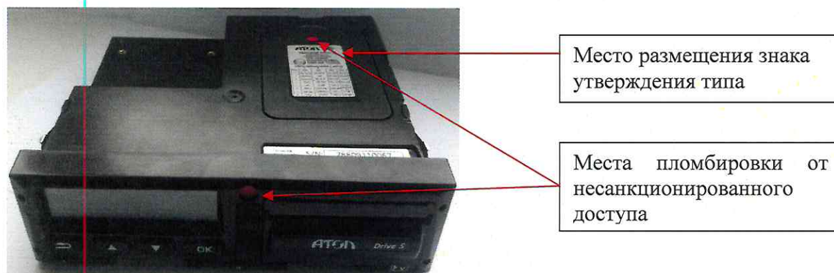
Рисунок 2 – Место размещения знака утверждения типа и схема пломбировки от несанкционированного доступа
